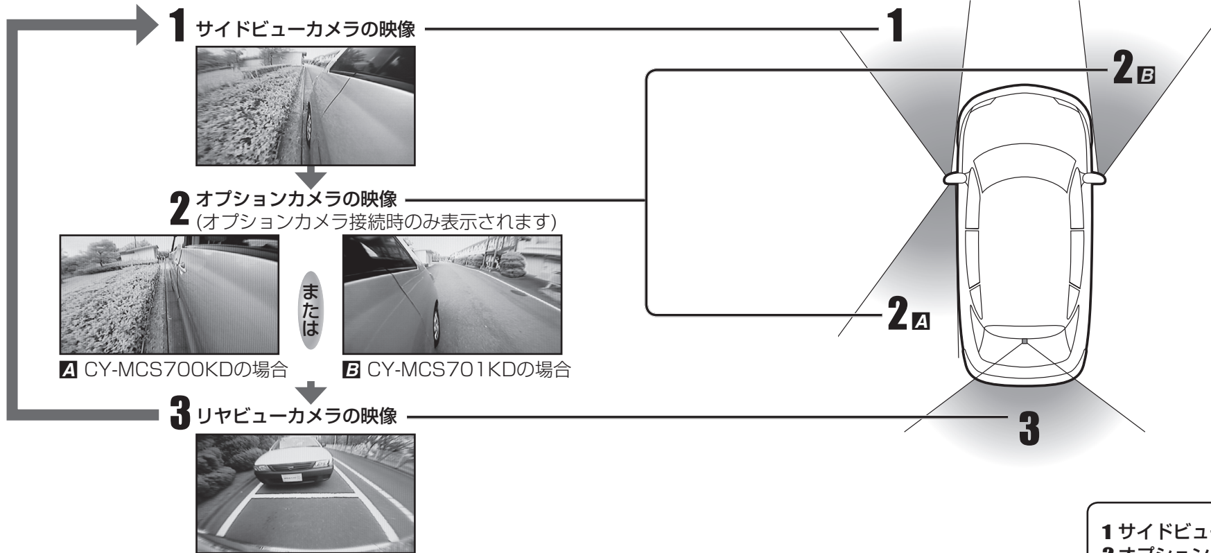
各カメラの取り付け位置と視野角
