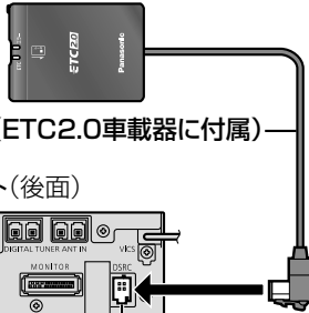
ETC2.0車載器接続端子(DSRC)
