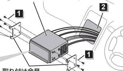
取り付け金具 (ブラケット)
