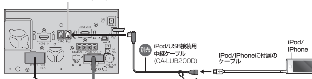
① ナビゲーションユニット(後面)
